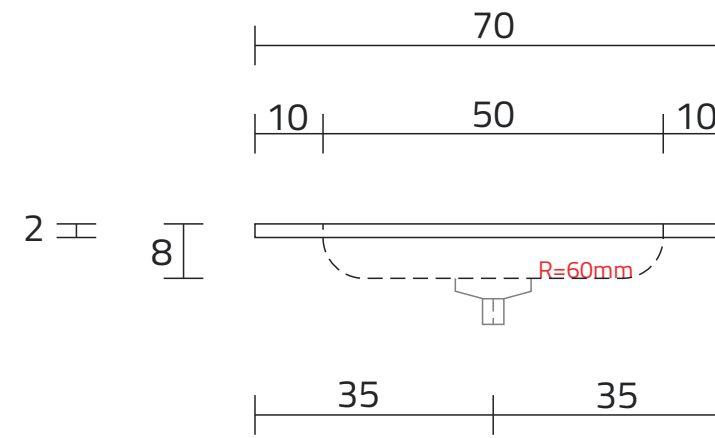
ROZMIESZCZENIE ODPŁYWU
