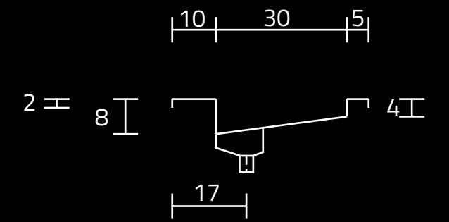
PRZEKRÓJ ,A'
