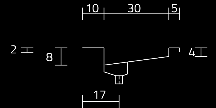
PRZEKRÓJ ,A'
