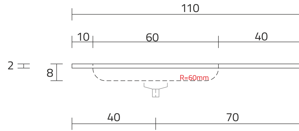
ROZMIESZCZENIE ODPŁYWU
