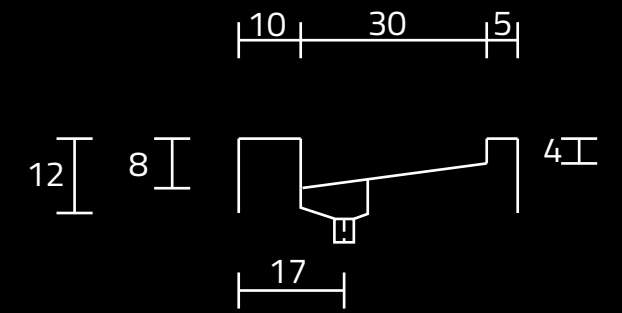
PRZEKRÓJ ,A'
